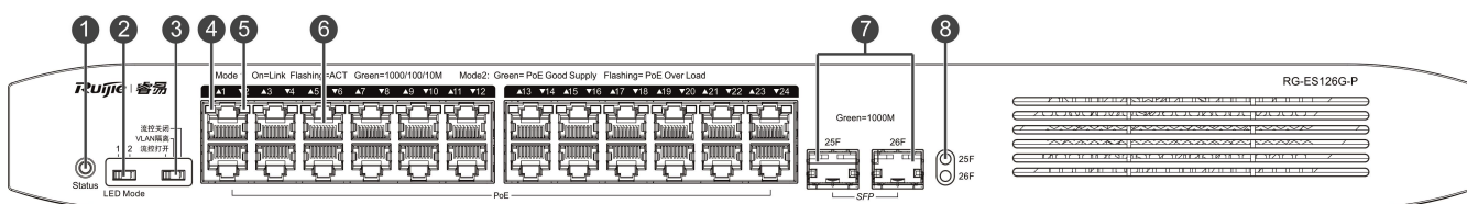
图 1-5 RG-ES126G-P 前面板图
