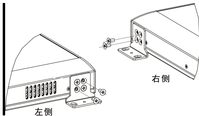
图 3-5 24 口设备挂壁式挂耳安装示意图一
