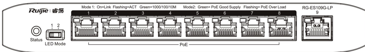
图 1-1 RG-ES109G-LP 产品外观图
