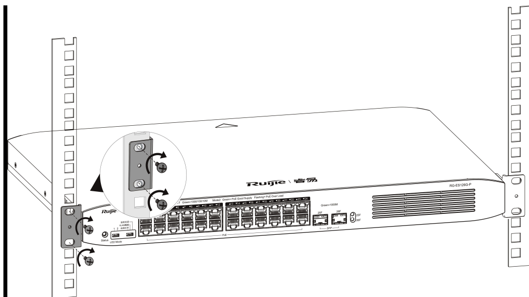
图 3-3 设备机柜式挂耳安装示意图三
