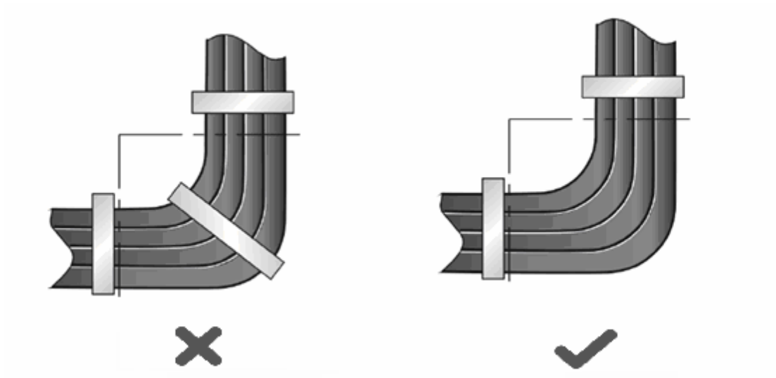
图 D-3 电缆捆扎示意图（三）
