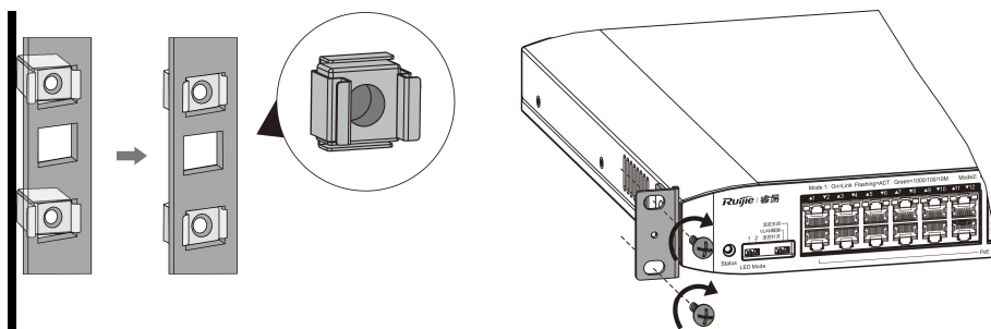
图 3-3 设备机柜式挂耳安装示意图三
