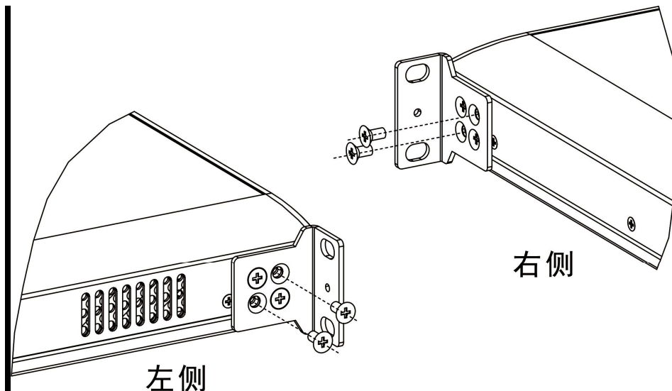
图 3-1 设备机柜式挂耳安装示意图一
